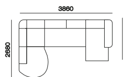
Бл-1у(850)-У-3у(1700)-К(850)
