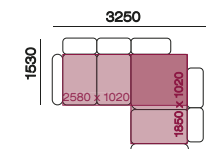
Бл-1у(700)-1у(700)-У-1у(700)-Бп
