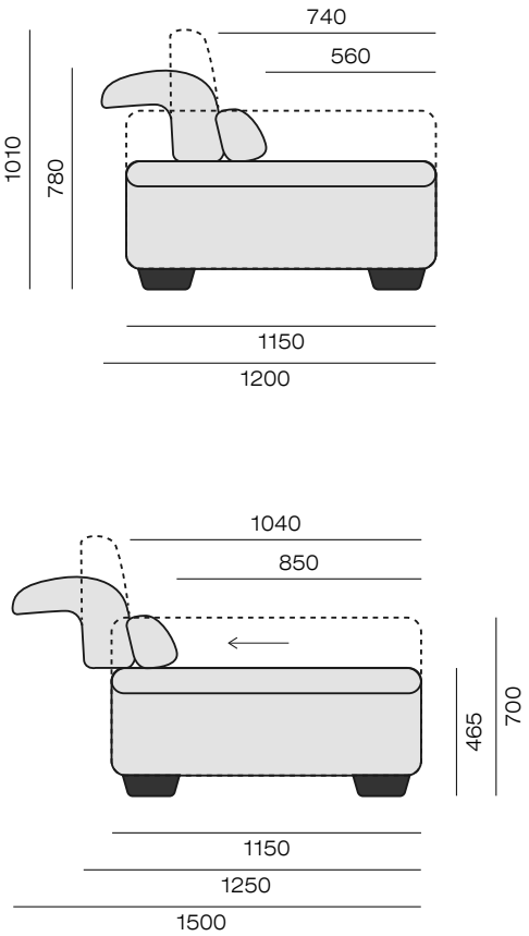
Диван сложен
