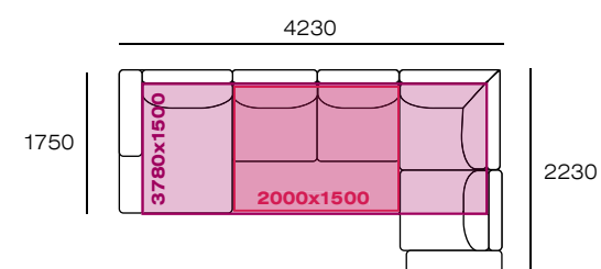
Б1л-К(Б)(1000)-2ру(2000)-У-1яу(1000)-Б1п
