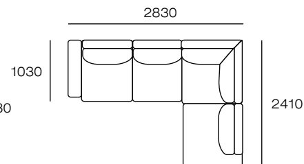
Б1л-2ру(1600)-У-1яу(Б)
