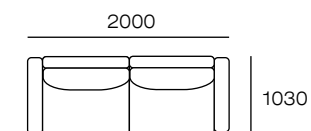
Б1л-2ру(1600)-Б1п Б1л-2у(1600)-Б1п*
