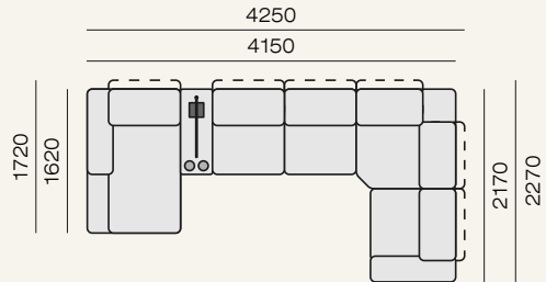
К(Т)(левый)-2у(Т)(барL)Э- У(Т)-1у(Т)(правый)-Бп
