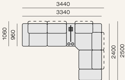
Бл-2у(Т)(бар)Э(левый)- У(Т)-1уБ(Т)(правый)
