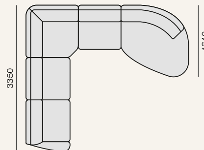
Бл-2у(1900)-У1-1у(950)-1уБ
