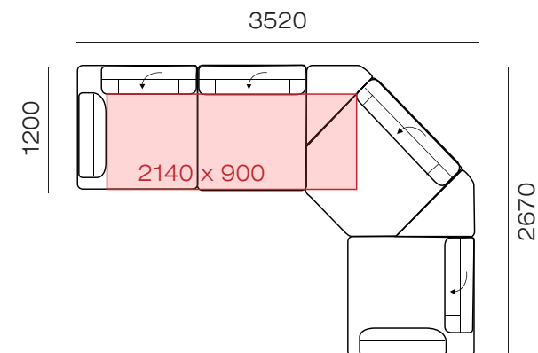
Бл-1у(850)-1у(850)-У-1у(850)-Бп
