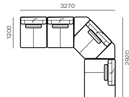
1у(850)-1у(850)-У-1уб(850)
