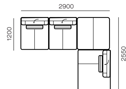
1у(850)-1у(850)-П-1уб(850)
