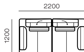
Бл-1у(850)-1у(850)-Бп
