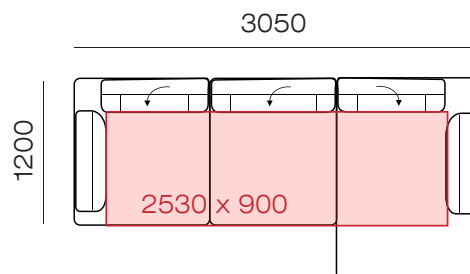
Бл-1у(850)-1у(850)-К(850)-Бп
