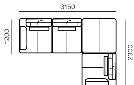
Бл-1у(850)-1у(850)-П-1у(850)-Бп
