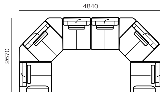
Бл-1у(850)-У-1у(850)-1у(850)-У-1у(850)-Бп
